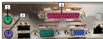
Figura 2(c) - Conectores da placa-mãe
